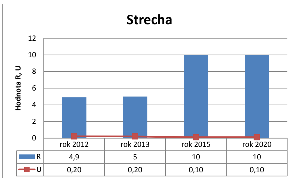
Obrázok 45: Strecha R a U
