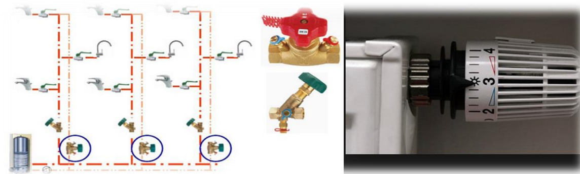
Obrázok 42: Hydraulické vyregulovanie TV, komponenty a termostatická hlavica
