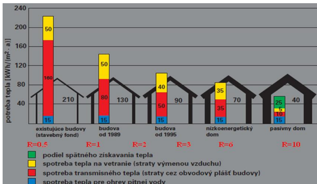
Obrázok 48: Spotreba energie v kWh/ 1m²/rok podľa R objektu
